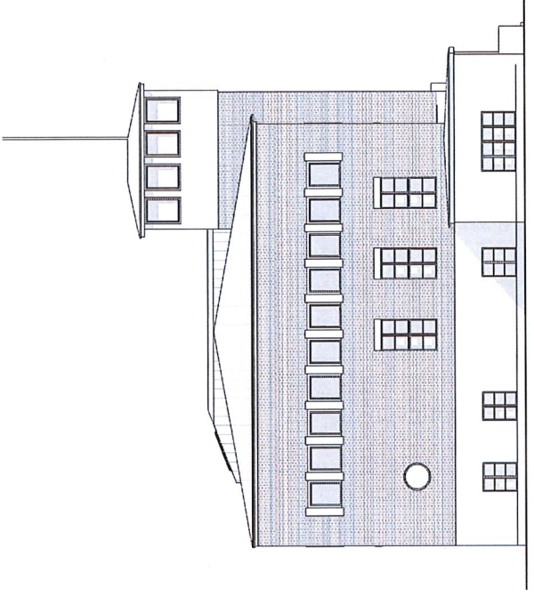
FASAD MOT SÖDER
